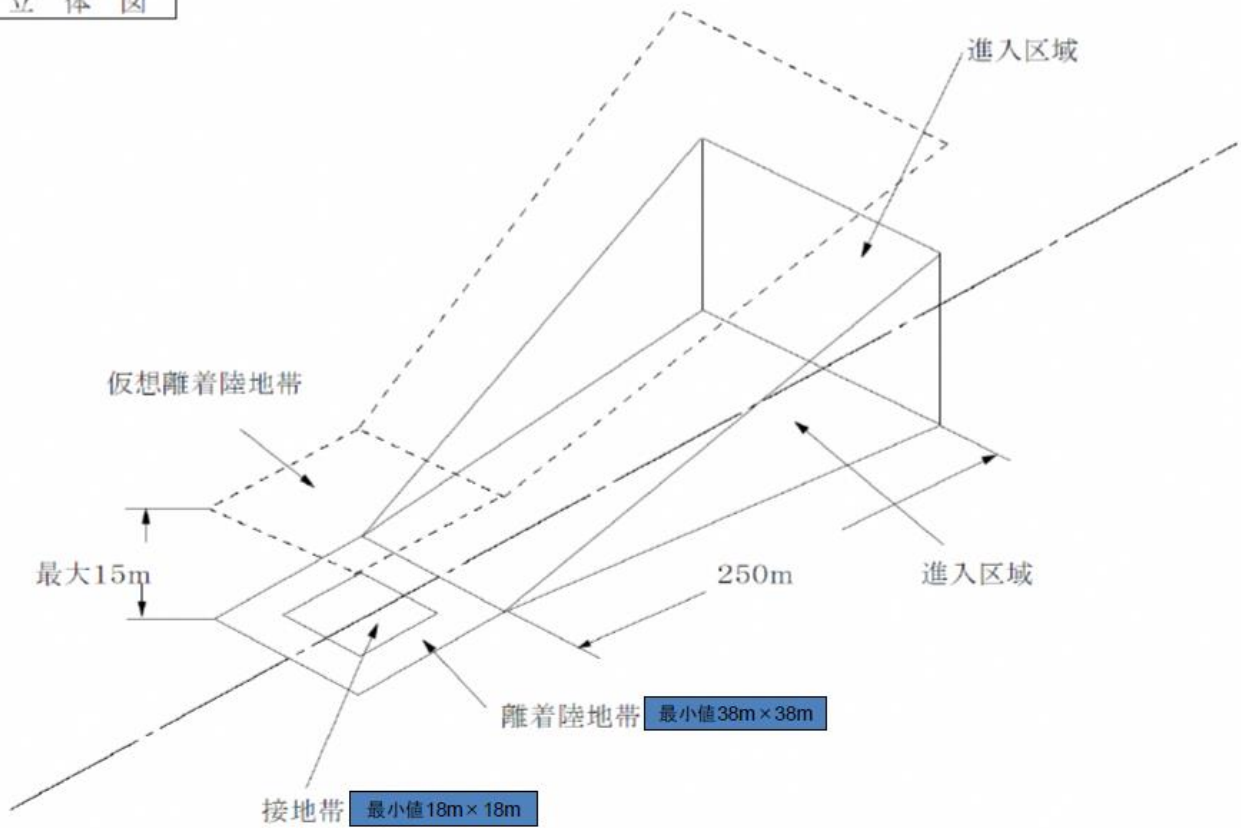
立体図
