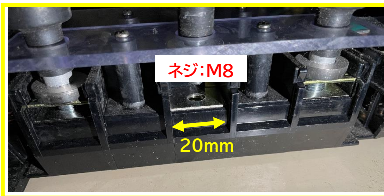
動力端子盤を下から覗き込んだ写真
