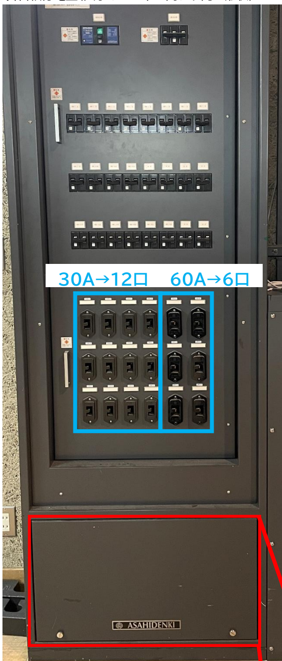
舞台袖分電盤(大小ホール下上問わず同一形状)
