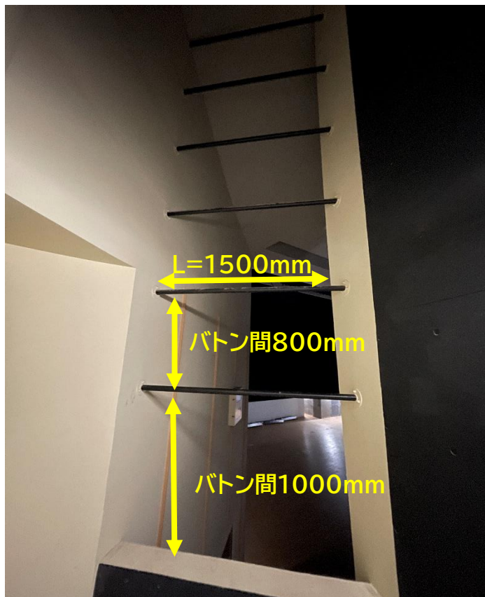
大ホールFS(下段)
